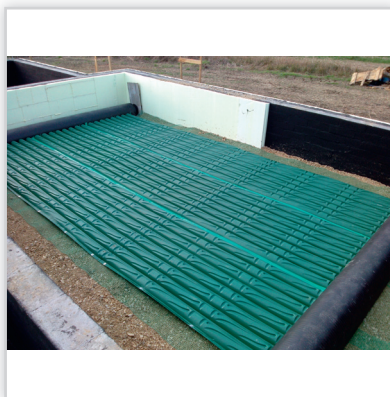
Gruntowy wymiennik ciepła GEOSTRONG – w fundamentach. GWC bezprzeponowy modułowy. Przepływ powietrza turbulentny, wymiana ciepła ze wszystkich stron GWC. Wytrzymałość na nacisk z góry: 460 t/m 2 . Zastosowanie: w wentylacji mechanicznej we współpracy z rekuperatorem w domach jednorodzinnych, wielorodzinnych i przemysł. Możliwość wykonania GWC o każdej wielkości przepływu powietrza. Możliwość samodzielnego montażu.
