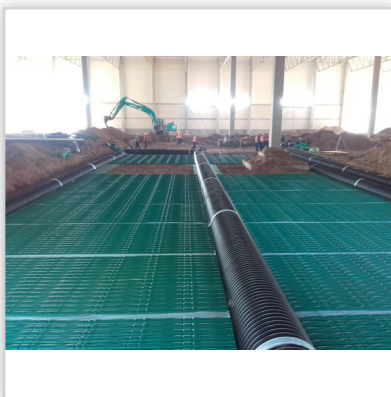
Gruntowy wymiennik ciepła GEOSTRONG – dla hali produkcyjnej. GWC bezprzeponowy modułowy. Przepływ powietrza turbulentny, wymiana ciepła ze wszystkich stron GWC. Wytrzymałość na nacisk z góry: 460 t/m 2 . Zastosowanie: w wentylacji mechanicznej we współpracy z rekuperatorem w obiektach użyteczności publicznej, pawilonach, magazynach, restauracjach. Możliwość wykonania GWC o każdej wielkości przepływu powietrza. Możliwość samodzielnego montażu.
